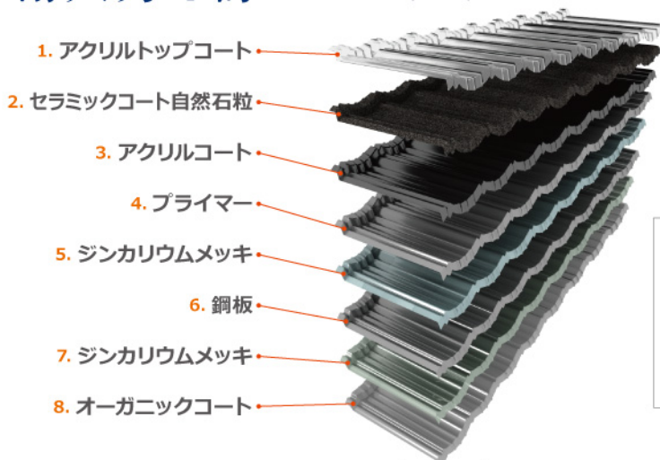
スカイメタルルーフ構造図
